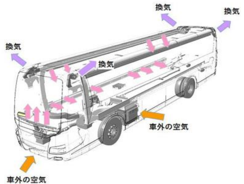
大型観光バス・床下A/Cタイプ
